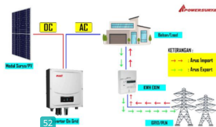
Gambar 2. Pembangkit Listrik Tenaga Surya[10]
