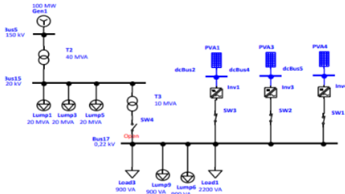
Gambar 3. Simulasi Aliran Daya Menggunakan Etap 4 Penulisan Laporan
