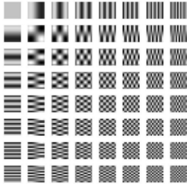
Gambar 1 dasar DCT lengkap ukuran N = 8
