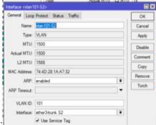
Gambar 10. Konfigurasi Sub-Interface VLAN 101- Trunk
